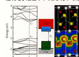
LaCuOSの2次元電子構造。CuS層(右図の赤い部分)に正孔が閉じ込められている。
