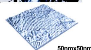
コンビナトリアルPLD表面解析複合装置：パルスレーザー堆積とSTMやLEED、AES分光装置とのin situシステムと二酸化チタンナノターゼ薄膜表面の原子分解能STM像
