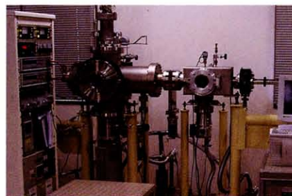
固体からの真空中への負イオン発生と照射評価システム
