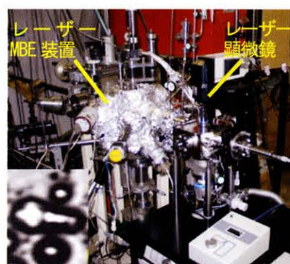
フラックスエピタキシー-レーザー顕微鏡複合装置：セラミックスの固液界面を利用した真空薄膜製造装置挿入図：BiOxの液滴のその場レーザー顕微鏡観察
