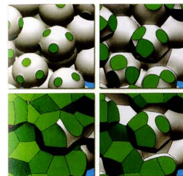
焼結プロセスの3次元シミュレーション(2006)
