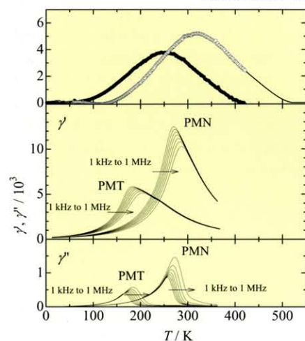
リラクサーにおける強誘電ナドメインの生成による過剰熱容量と誘電率
