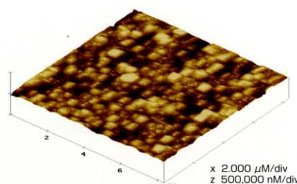
フロー式水熱電気化学セルを用いてBa溶液中(150℃, 1h)で生成した結晶性BaTiO 3 膜
