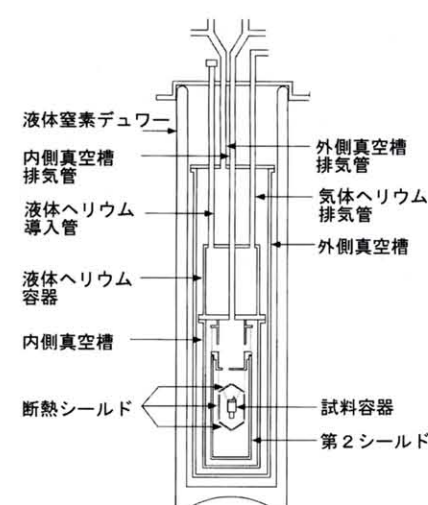
超高精度断熱型熱量計
