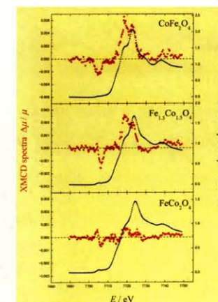
フェライトやコバルタイトでの磁気吸収
