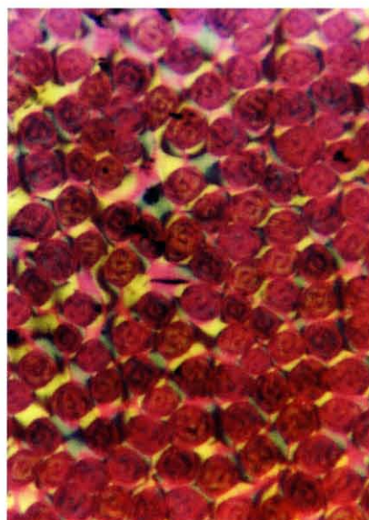
C/C複合材料の偏光顕微鏡観察黒鉛構造の発達により光学異方性が生じる
