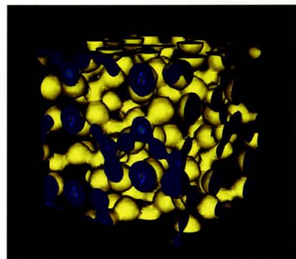
実測による、水素化物イオン \text{H}^- を包接する籠状格子の構造
