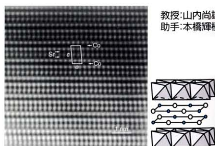
新規「ミスフィット」層状酸化物：[Sr 2 O 2-w ] 0.5 CoO 2 の高分解能電子顕微鏡像
