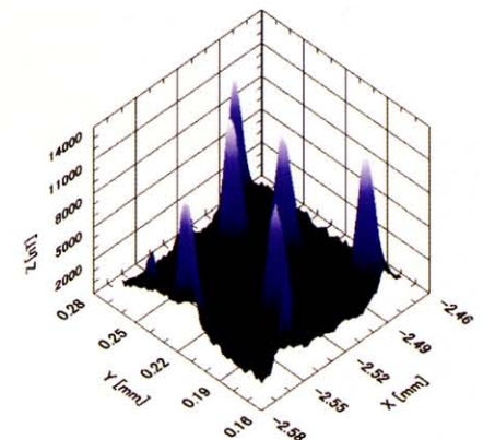
超伝導体にトラップされた地磁気
