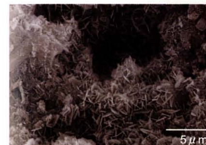
150°Cの低温下での水熱合成に成功したバモライト ( [\text{Ca}_4(\text{Si}_3\text{O}_9\text{H})_2]\text{Ca} \cdot 4\text{H}_2\text{O} )
