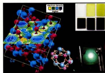
(左)エレクトライドC12A7: \text{e}^- の結晶構造と電子分布。 (中央) ナノ籠構造(籠の内径は \sim 4\text{\AA} )。 (右上) 電子が生成する様子が色の变化でわかる。 (右下) 電界放射型発光デバイス。
