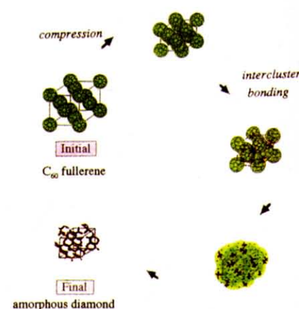
フラーレンの相転移を凍結したアモルファスダイヤモンド
