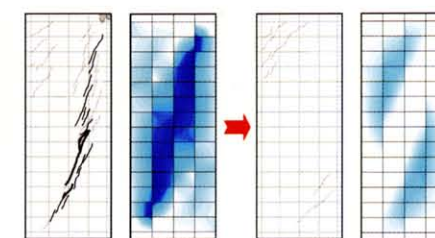
横方向プレストレスによるせん断ひび割れの抑制効果
