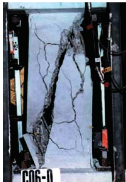
実験で再現した柱のせん断破壊 Experimental result
