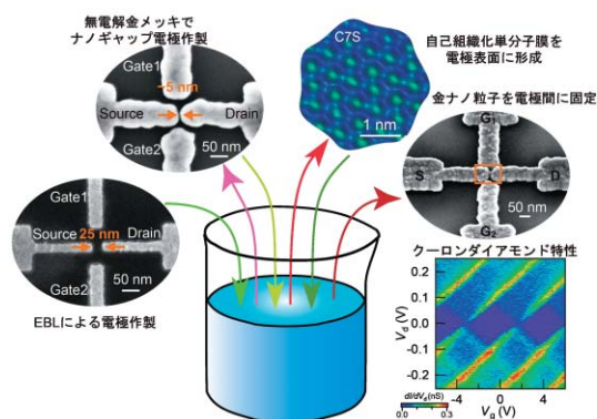
ボトムアップ手法により組み上げた単電子トランジスタとクーロンダイヤモンド特性 Chemically assembled single-electron transistor and Coulomb diamond characteristic.
