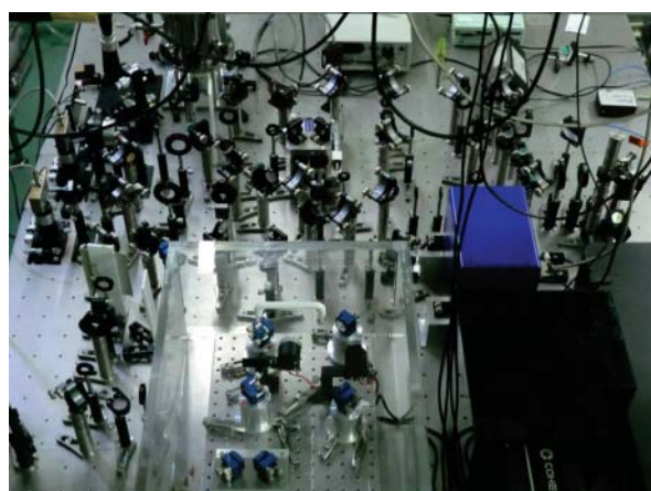
フェムト秒時間分解分光装置
