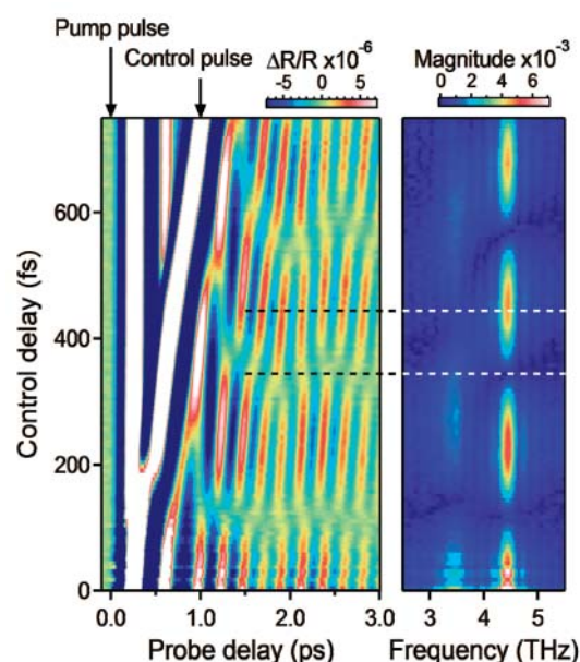
YBa 2 Cu 3 O 7-d のコヒーレントフォノン制御
